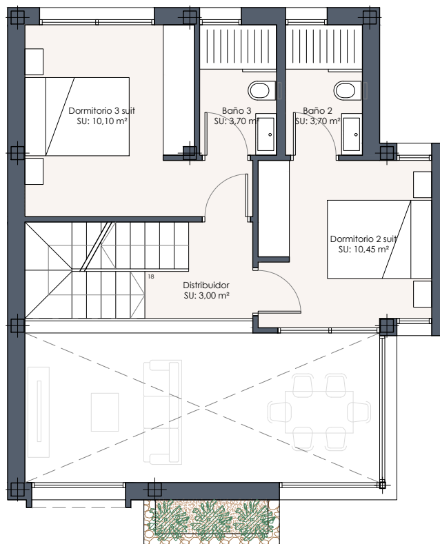
PLANTA PRIMERA
