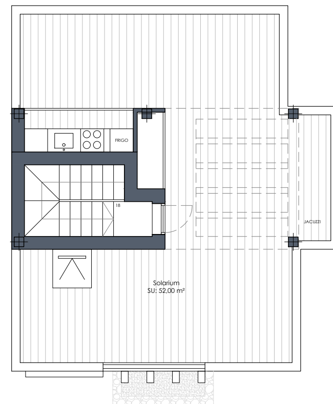
PLANTA CUBIERTA
